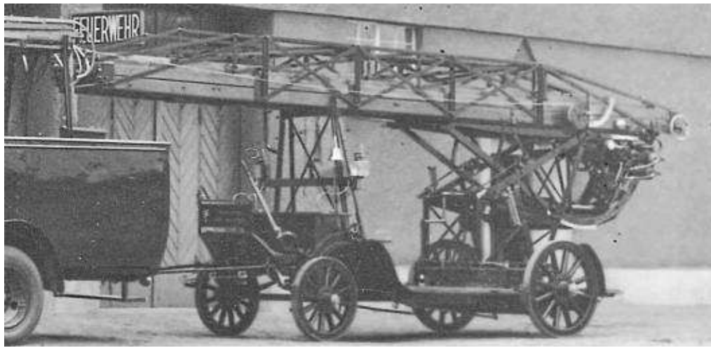
Diese Vierradleiter aus dem Jahr 1932 war einst ein gängiges Einsatzfahrzeug.
